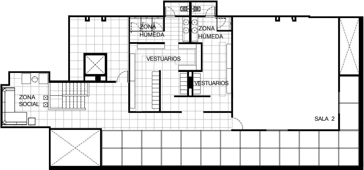
Planta Superior
