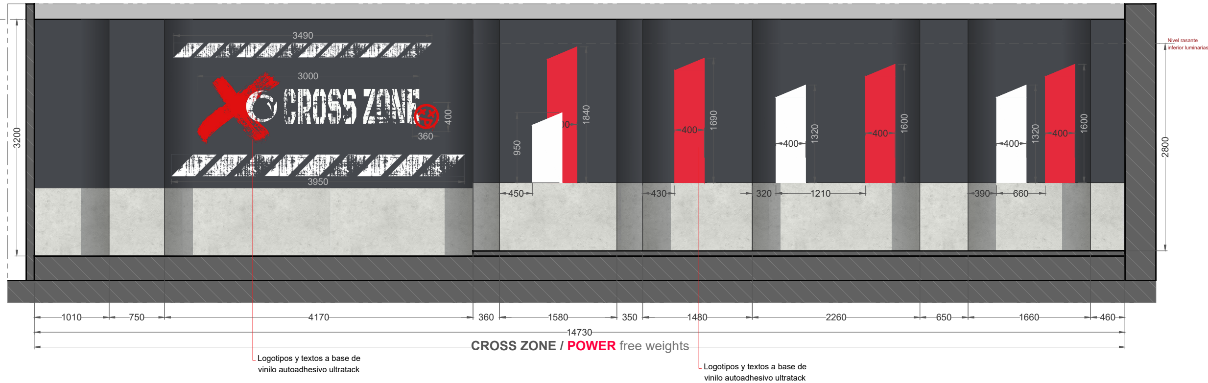
Alzado G | E: 1/50
