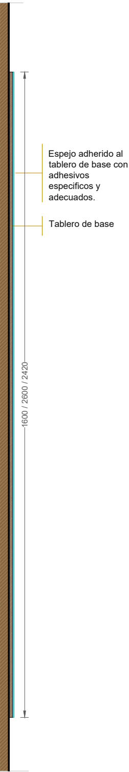
Sección espejos retranqueados | e: 1/15
