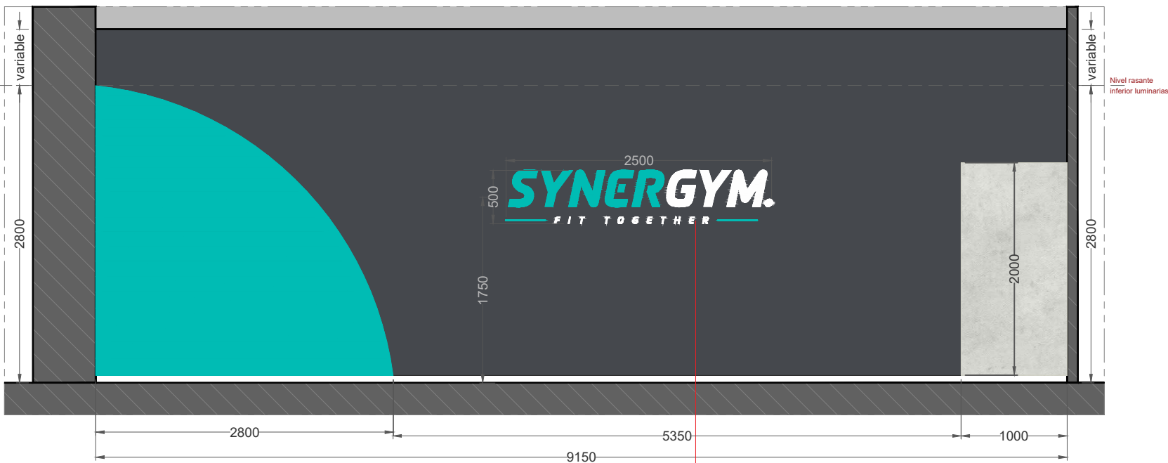
Alzado 4 | E: 1/50
