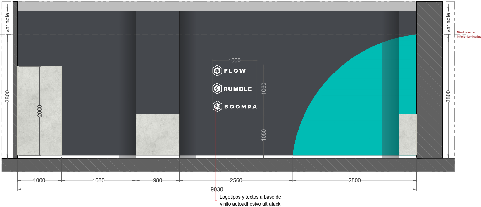
Alzado 2 | E: 1/50
