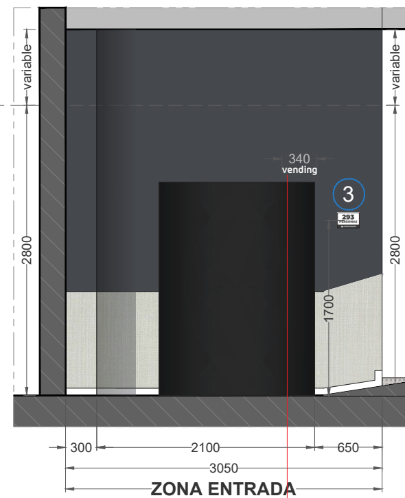
Alzado B | E: 1/50
