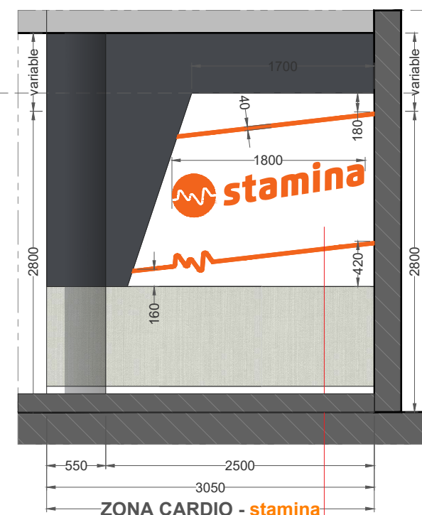
Alzado C | E: 1/50
