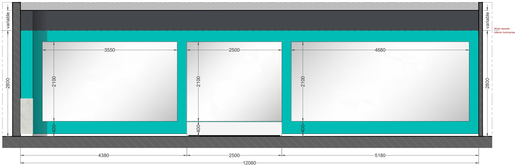
Alzado 3 | E: 1/50
