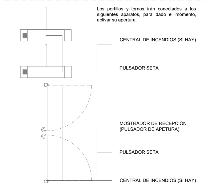
Esquema de funcionamiento tornos y portillo. Escala 1:50
