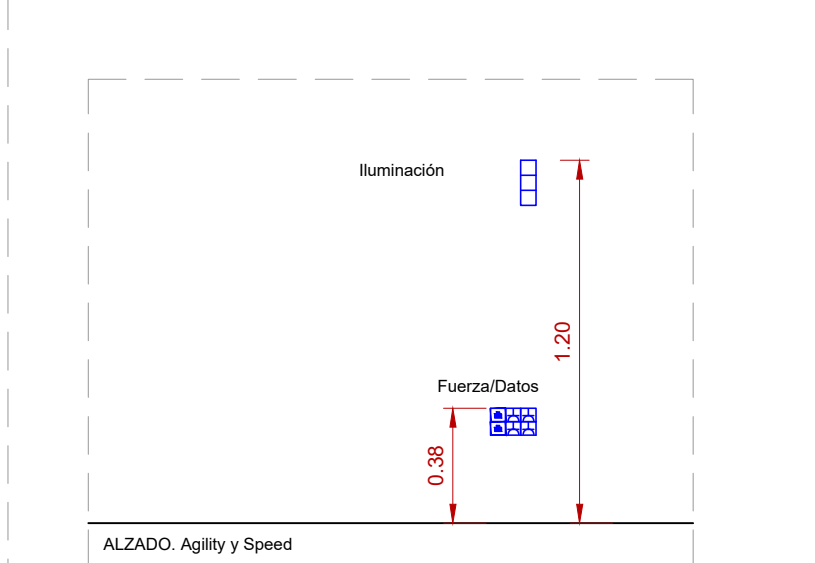
Detalle replanteo mecanismos. Escala 1:25
