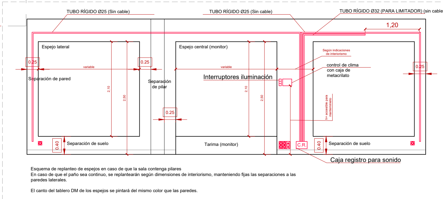
Detalle alzado clase de Agility. Escala 1:50
