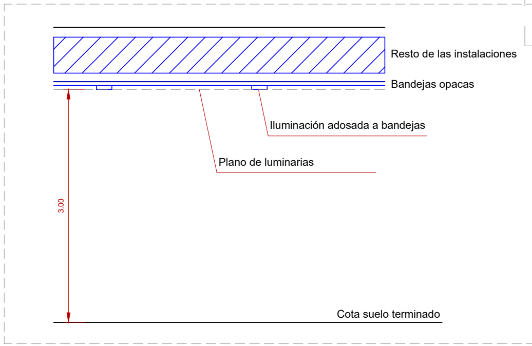
Detalle replanteo plano de iluminación. Escala 1:50
