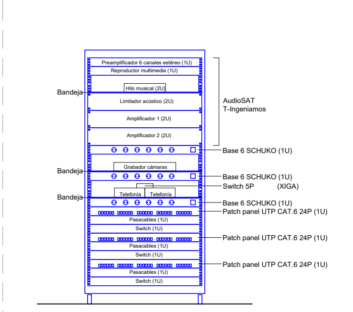
ESQUEMA DE RACK 19" 20U. Escala 1:15
