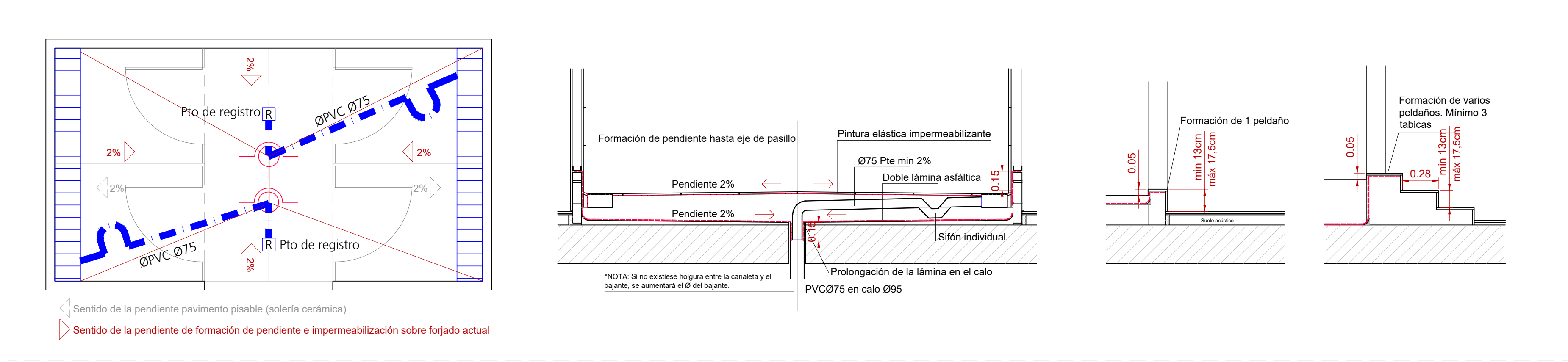
Detalle formación de pendiente en duchas un único calo para cada núcleo de duchas. Escala 1:25
