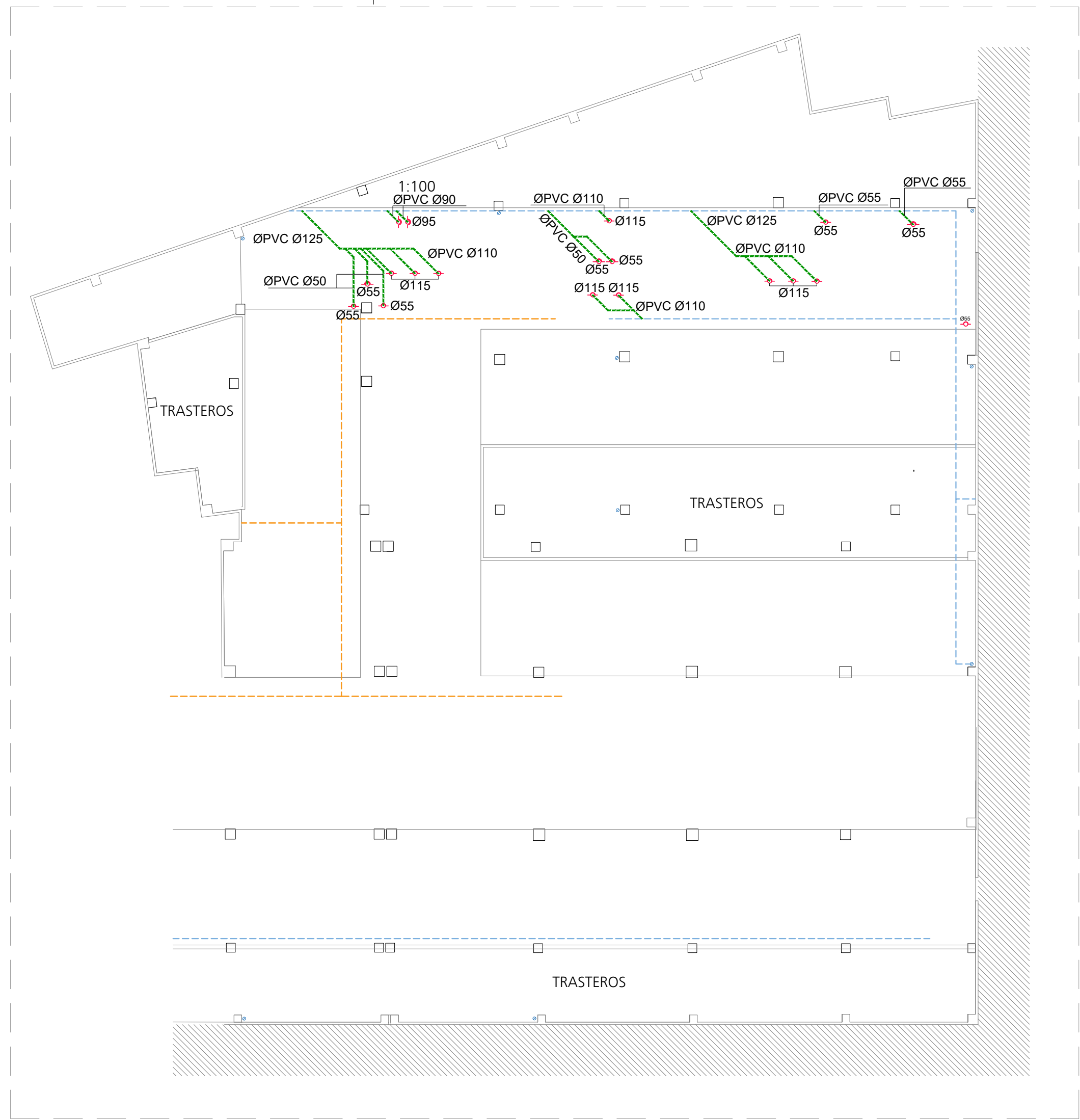
Planta sótano. Escala 1:150
